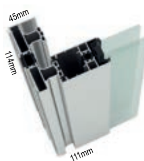
Sistema PL Système PL | PL System
