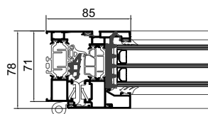
ST-Clássica | Classic | Classique
