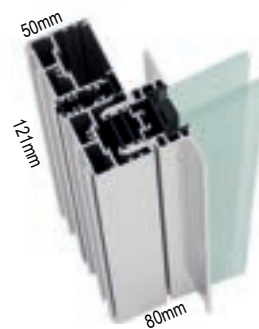
Sistema JE Système JE | JE System
