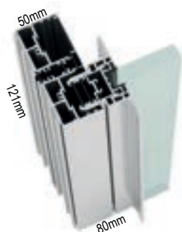
Sistema JT Système JT | JT System
