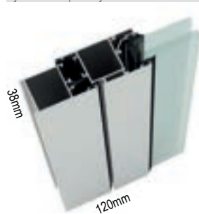
Sistema SB Système SB | SB System
