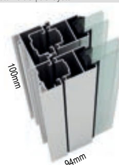
Sistema JG Système JG | JG System
