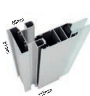
Sistema PS Système PS | PS System
