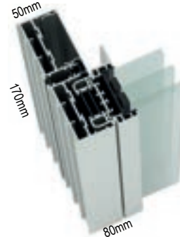
Sistema TL Système TL | TL System
