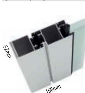
Sistema PS Système PS | PS System
