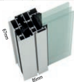
Sistema LT Système LT | LT System
