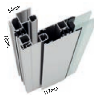
Sistema SP Système SP | SP System
