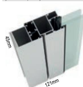
Sistema SA Système SA | SA System
