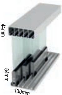
Sistema OR-PV - Portas de vidro de correr Système OR-PV - Portes coulissantes en verre OR-PV System - Sliding glass doors
