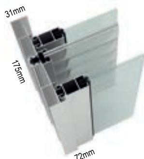
Sistema OS-P Système OS-P | OS-P System
