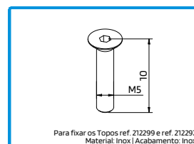
290107 PARAFUSO M5x10
