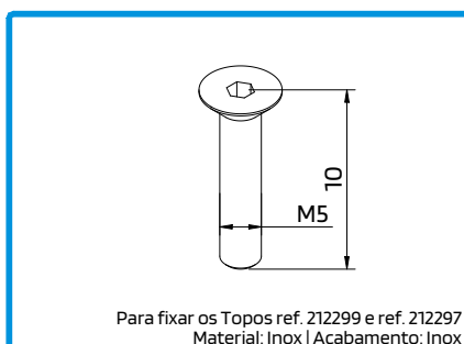
290107 PARAFUSO M5x10
