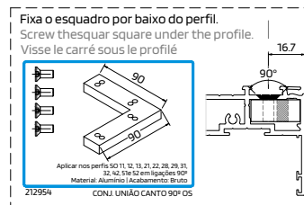
212954 CONJ. UNIÃO CANTO 90º OS
