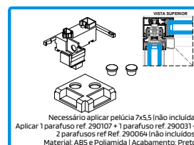
212299 CONJ. TOPOS SUP/INF SO 10 ESQUERDO PRT
