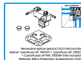
212297 CONJ. TOPOS SUP/INF SO 10 DIREITO PRT
